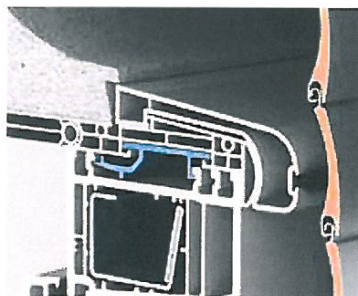
Beispiel mit blendrahmenspezifischem Anbindungsprofil bei KARO
