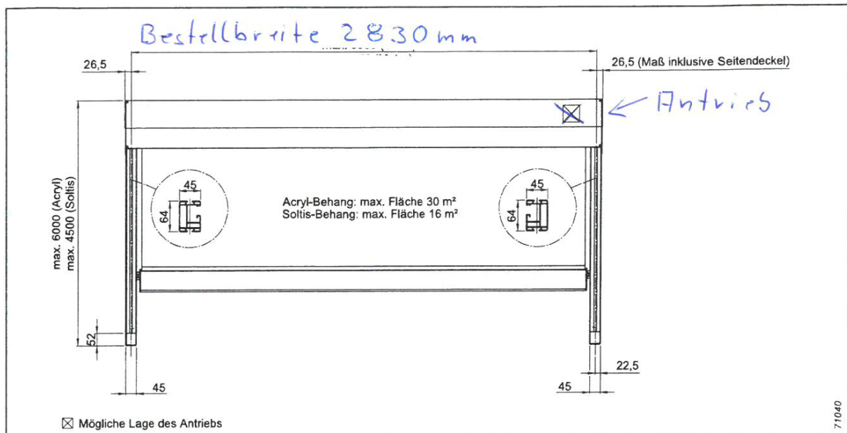
Abb. 332: Maßanleitung Einzelanlage
