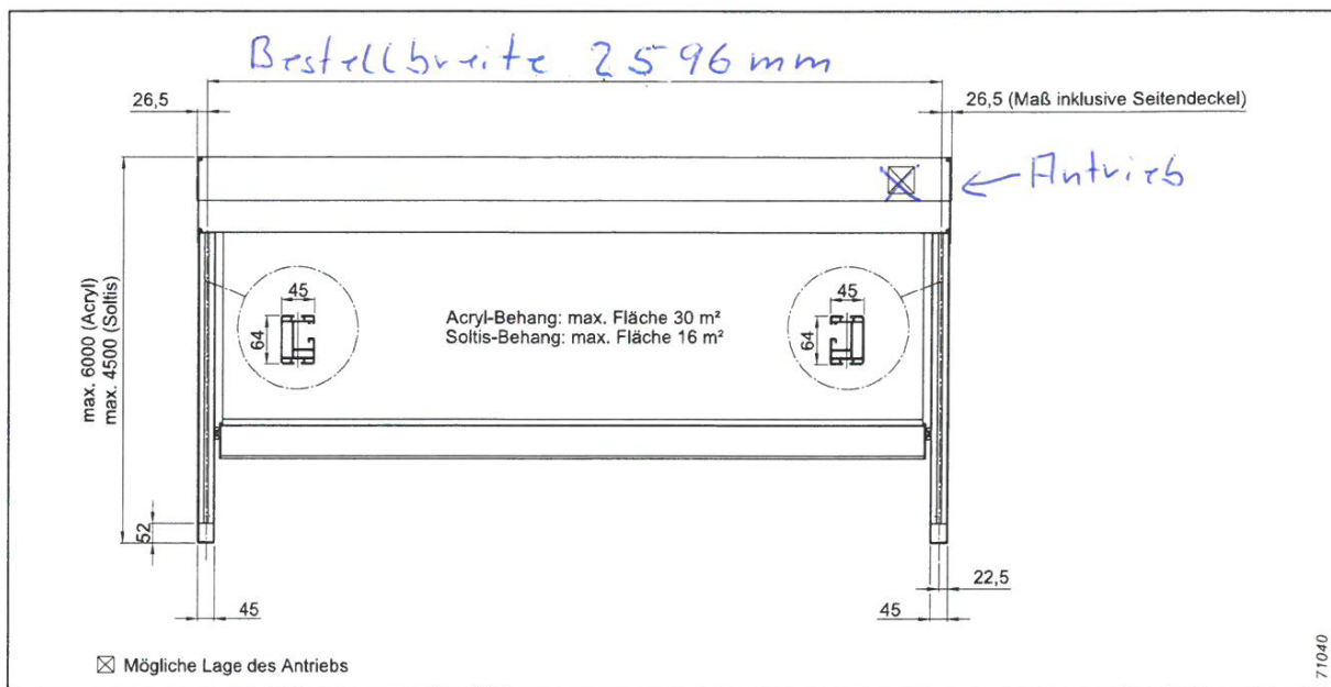
Abb. 332: Maßanleitung Einzelanlage
