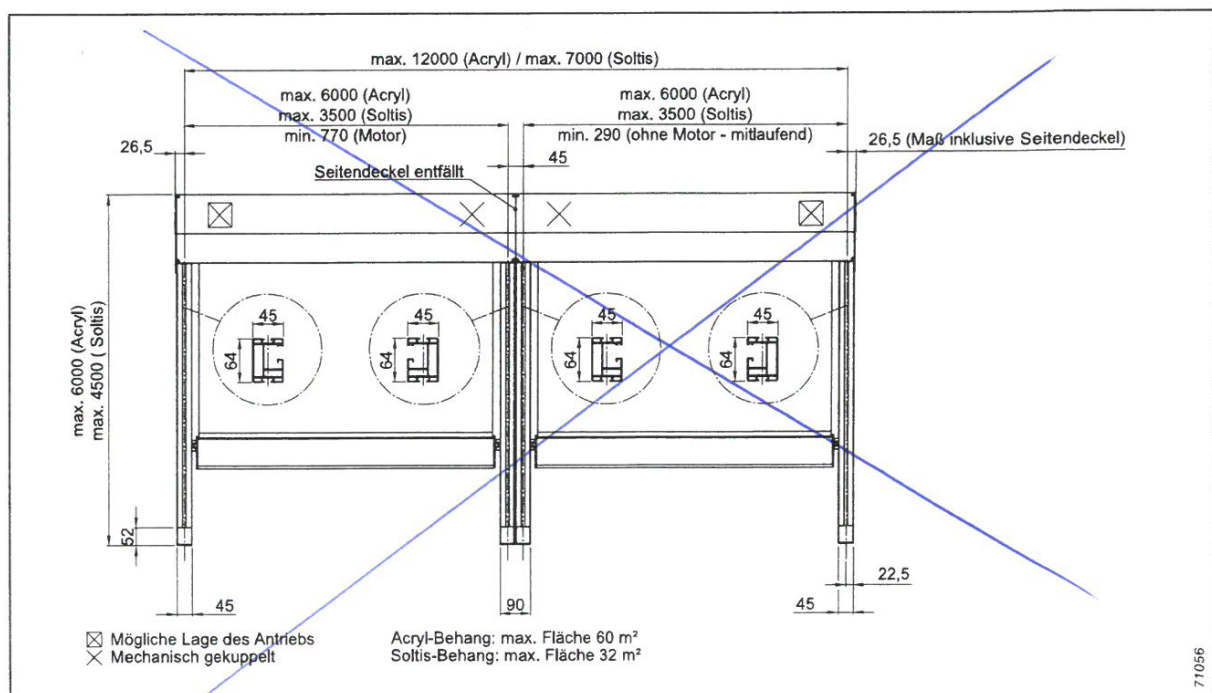
Abb. 333: Maßanleitung mechanisch gekuppelte Behänge
