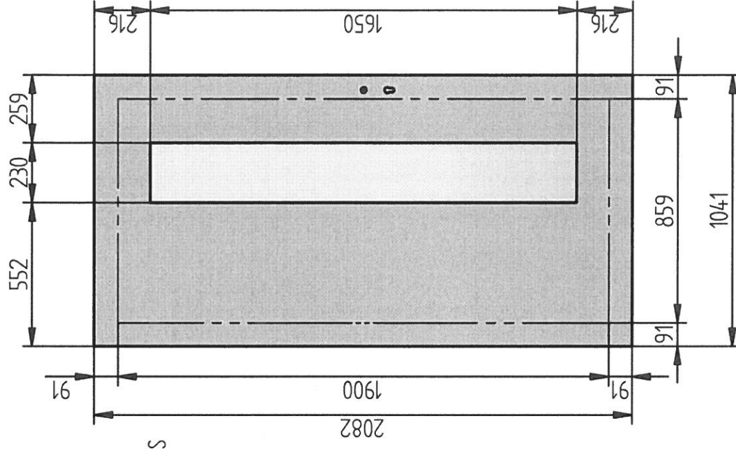
Innenansicht
