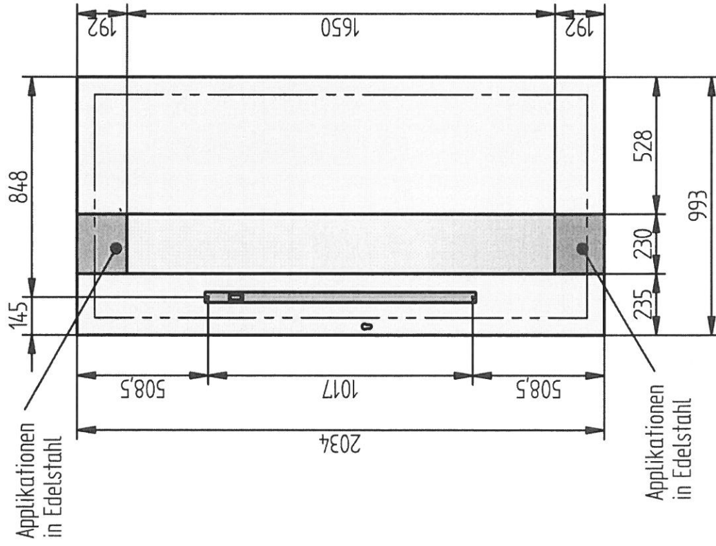
Außenansicht
