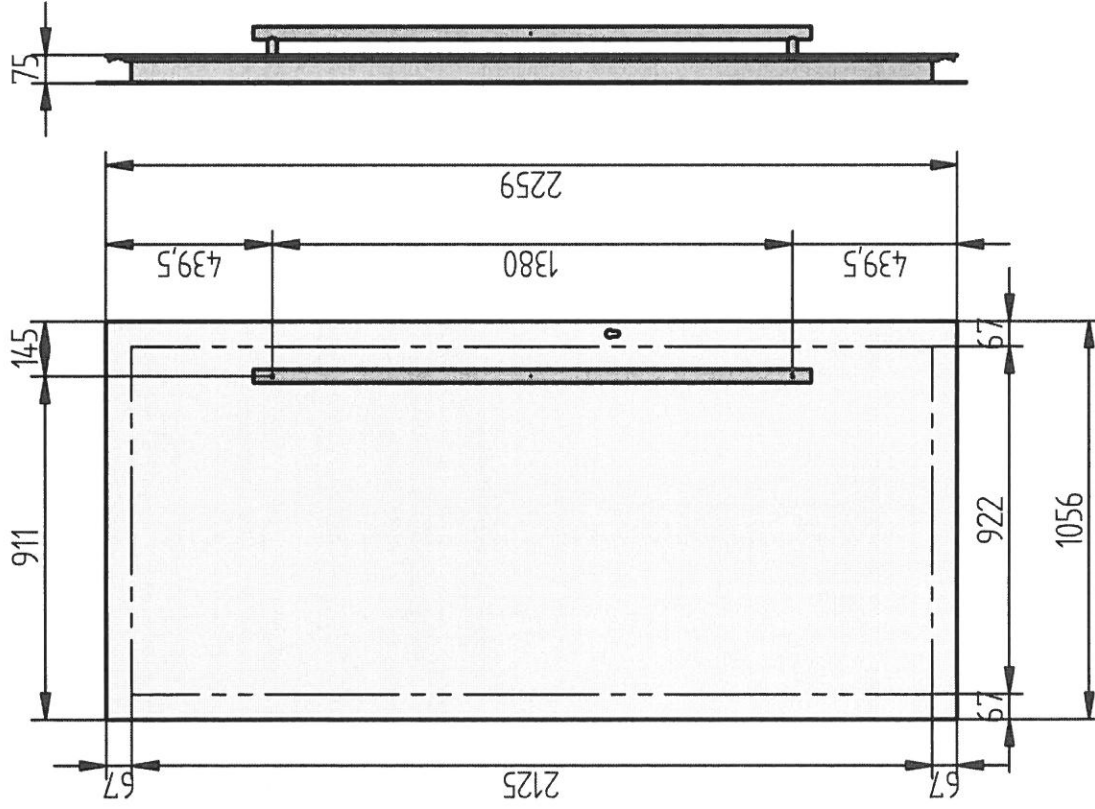
Aussenansicht
