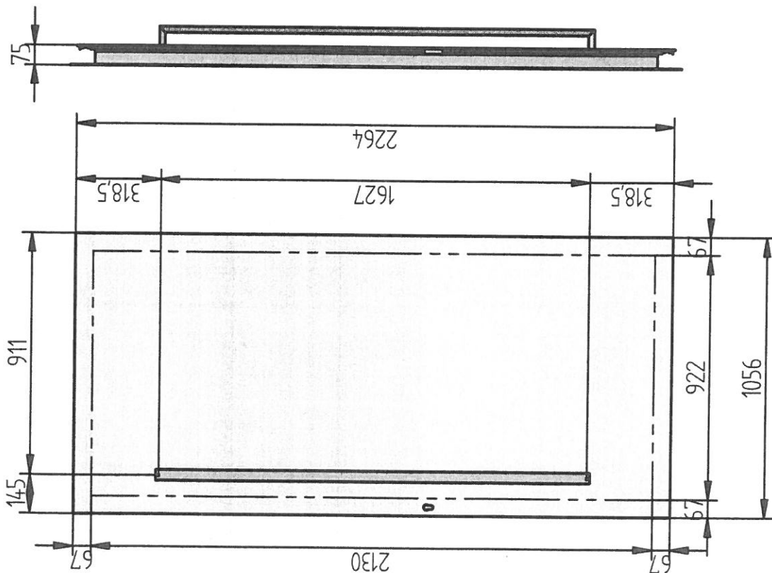
Aussenansicht
