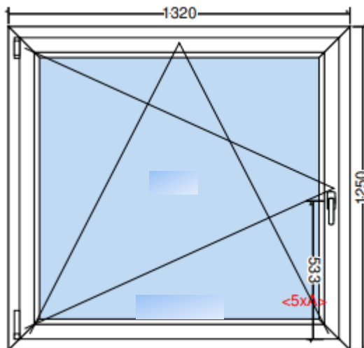
Innen Ansicht
