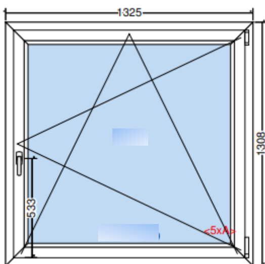
Innen Ansicht
