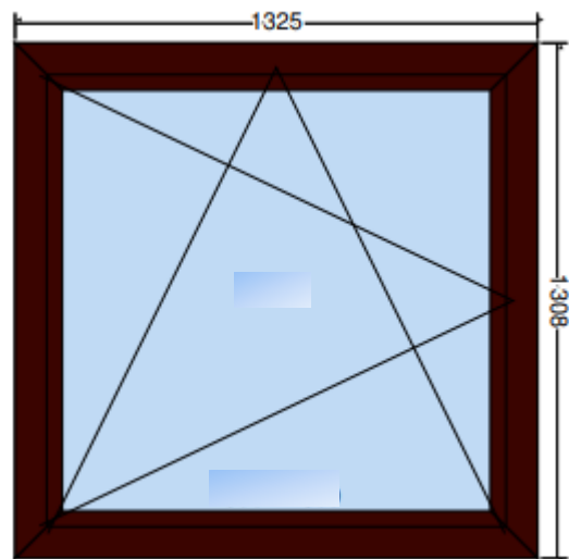
Aussen Ansicht
