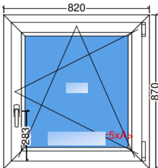
Innen Ansicht
