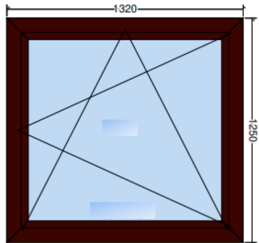
Aussen Ansicht
