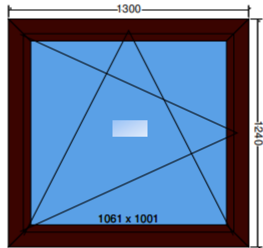
Aussen Ansicht
