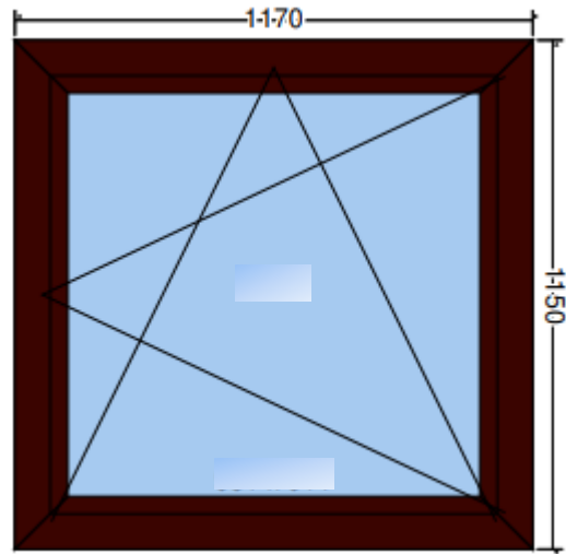
Aussen Ansicht
