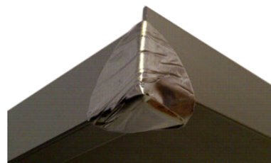
FBBPF Butyl-Eckabdichtung
