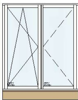
Internorm Holz/Alu Fenster Breite: 2070mm, Höhe: 2370mm, Breitenteilung: 1035/1035, Einbaufelder: SFG/SFS, Unterstück für 250 mm Fußbodenaufbau
