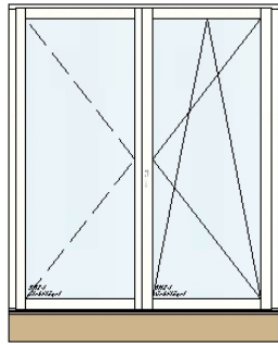
Einbaufelder: TSFS/TSFG Unterstück für 250 mm Fußbodenaufbau
