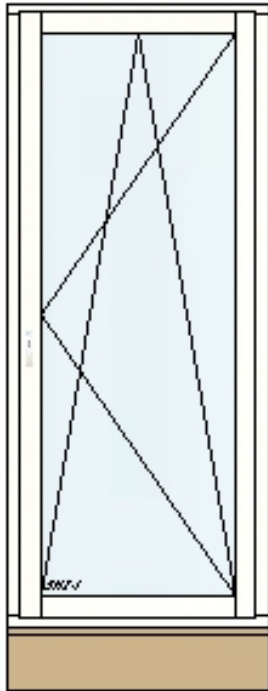
Internorm Holz/Alu Fenster Breite: 980mm, Höhe: 2370mm, Einbaufelder: SF, Unterstück für 250 mm Fußbodenaufbau
