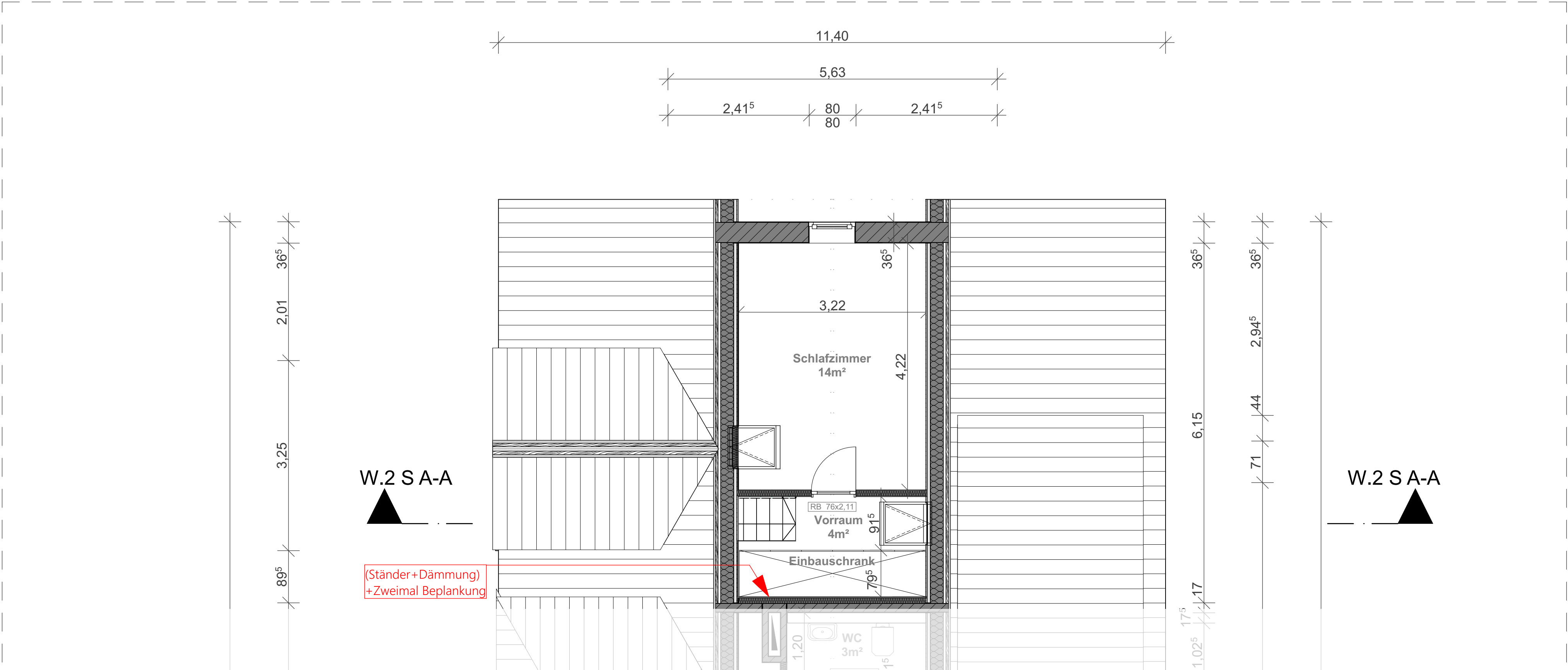
2. DG 1:50
