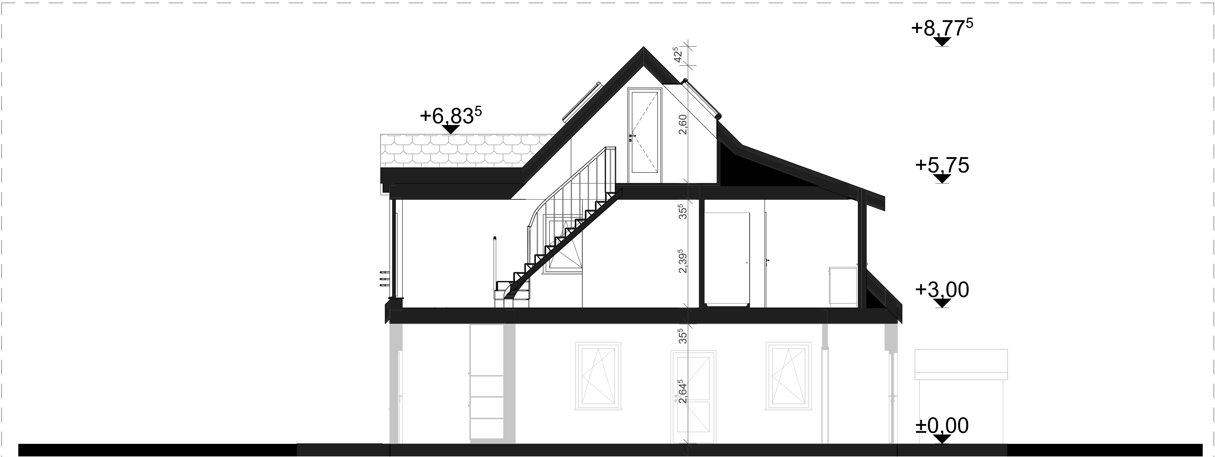
S A-A Schnitt A-A 1:50
