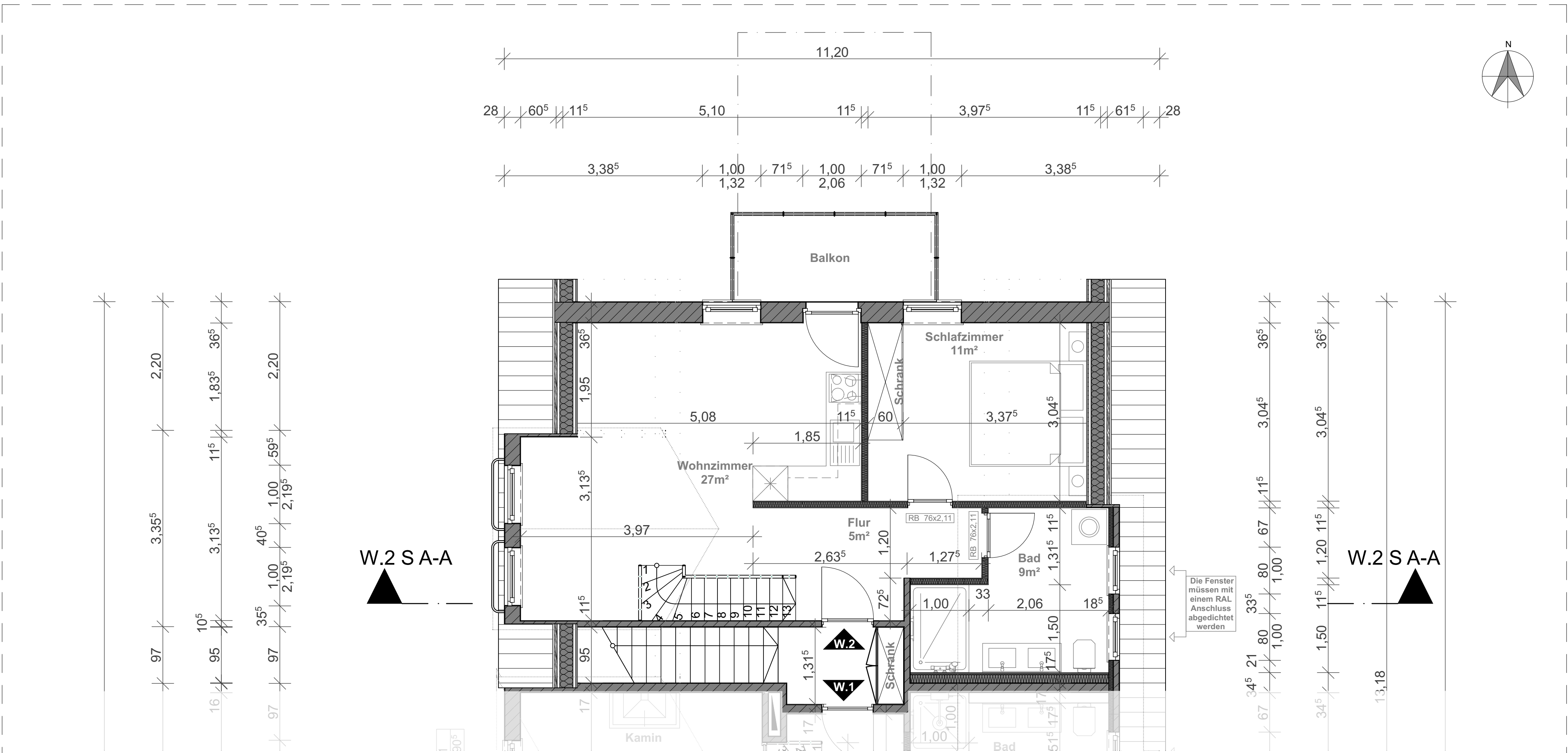
1. 1. OG 1:50
