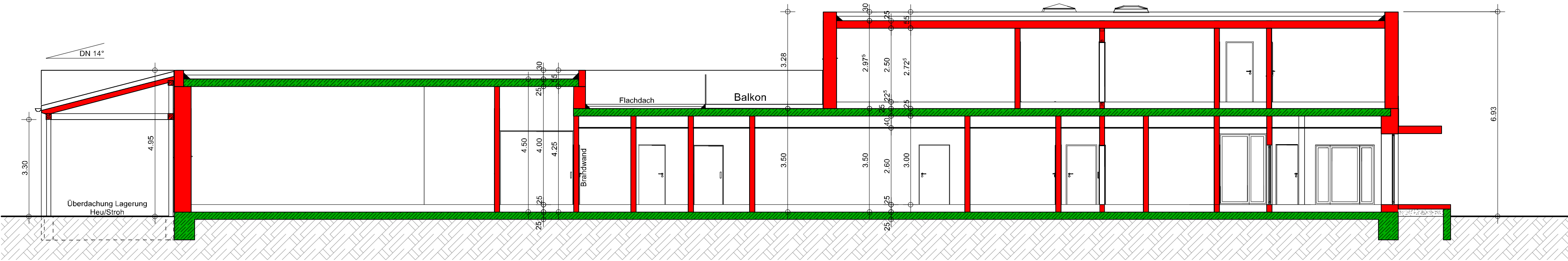
SCHNITT A-A
