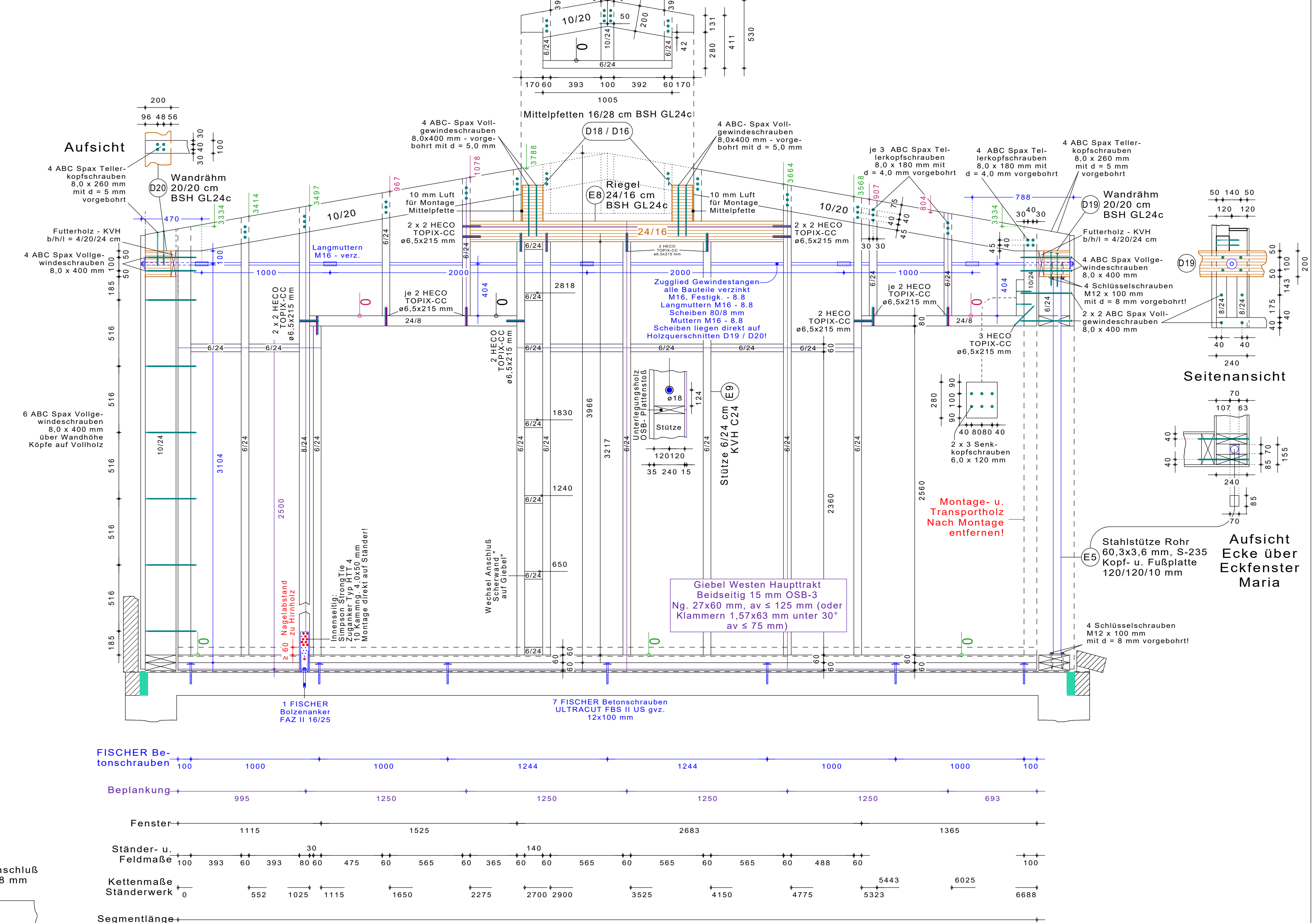
Giebel Haupttrakt - Westen
