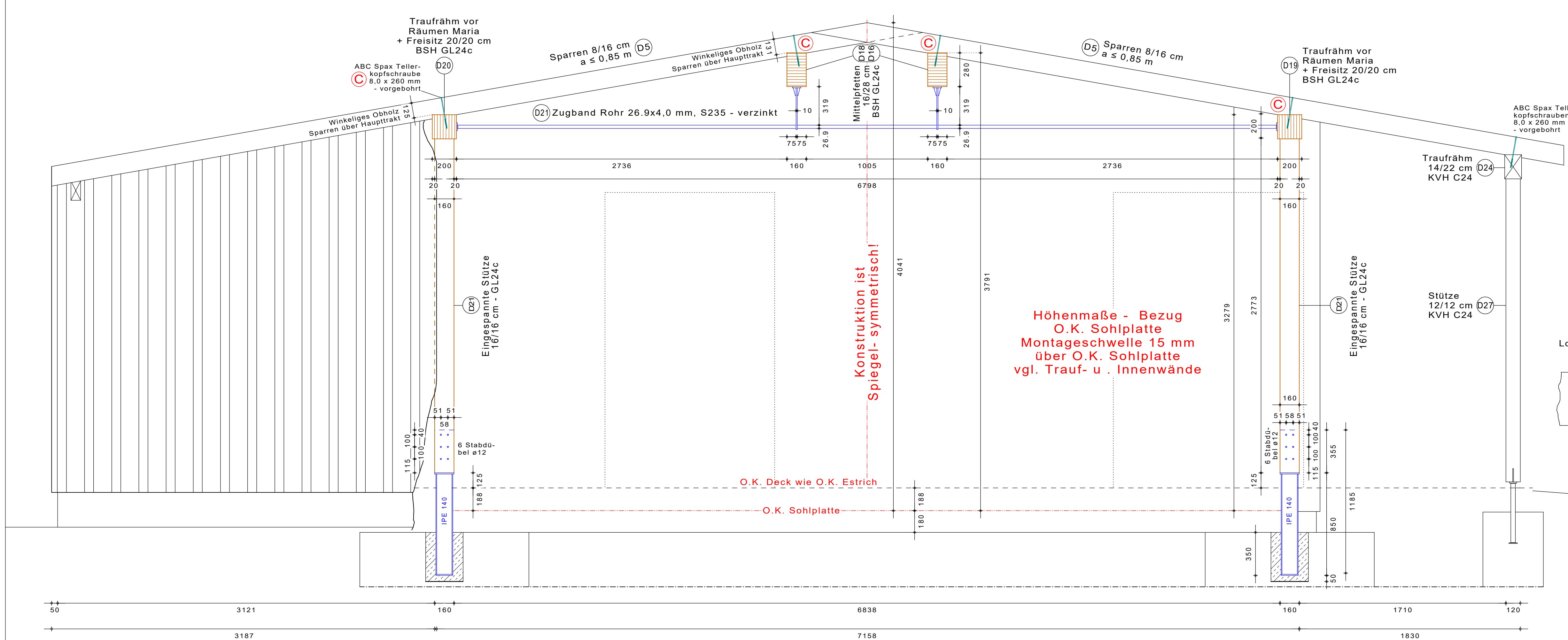
Pos D21 Eingespannte Stützen - Terrasse vor Räume Maria
