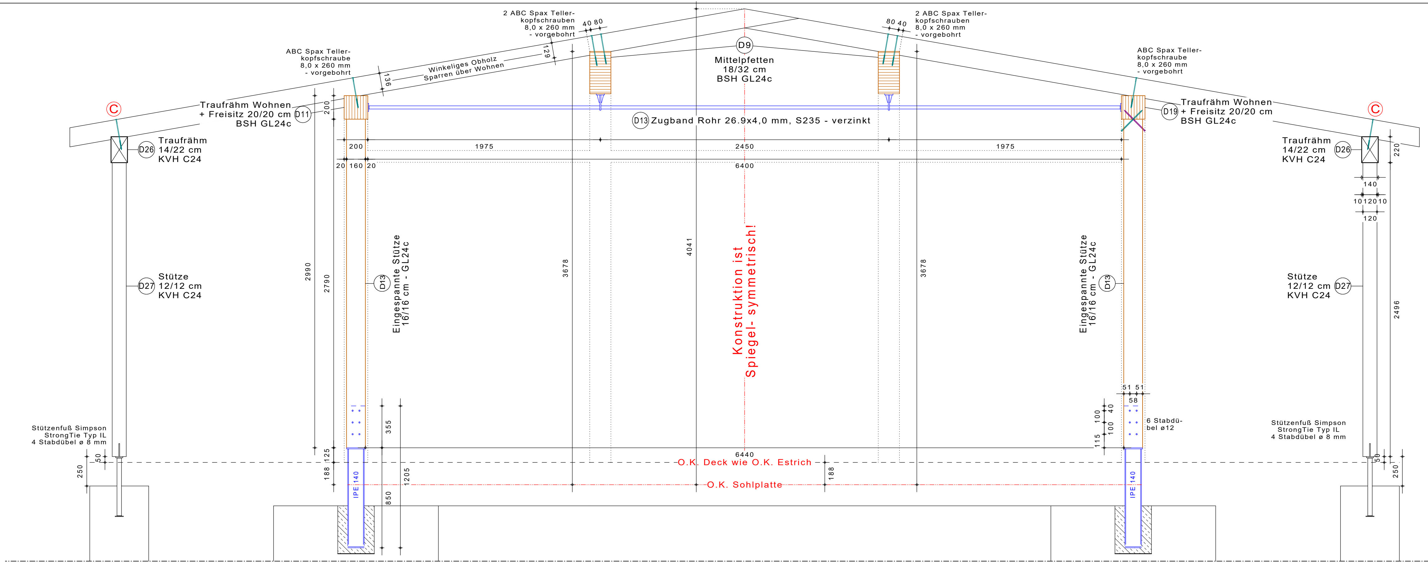
Pos D13 Eingespannte Stützen Terrasse vor Wohnen
