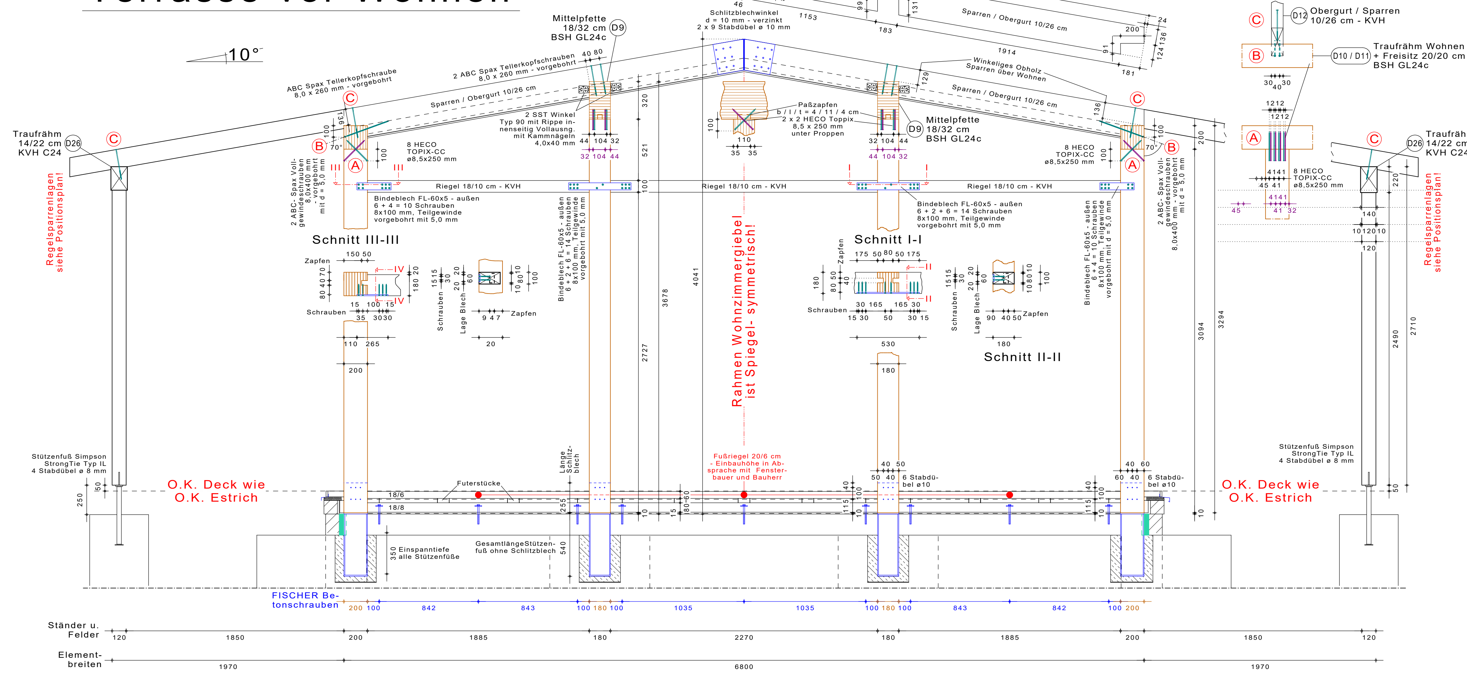
Pos D12 Giebelrahmen Wohnen
