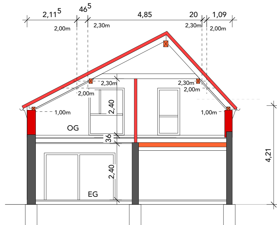
Schnitt AA
