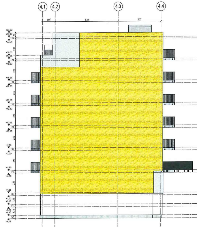
ANSICHT RECHTS
