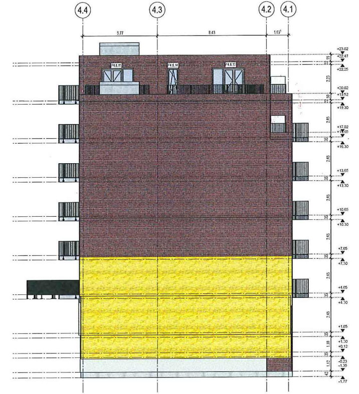
ANSICHT LINKS
