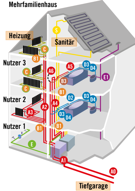
Mehrfamilienhaus
