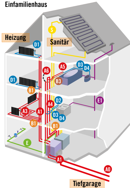
Einfamilienhaus
