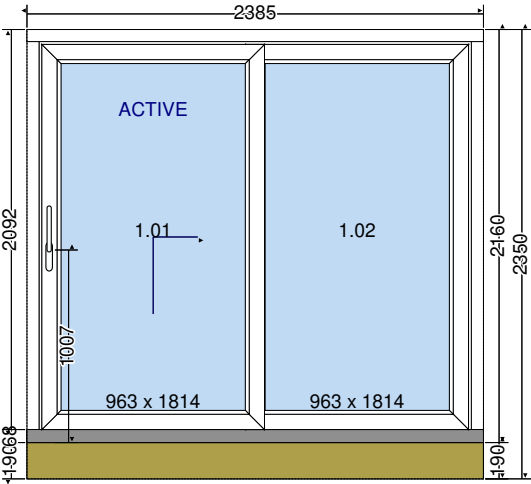
Innen Ansicht
