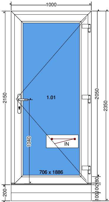
Innen Ansicht
