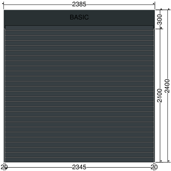
Innen Ansicht
