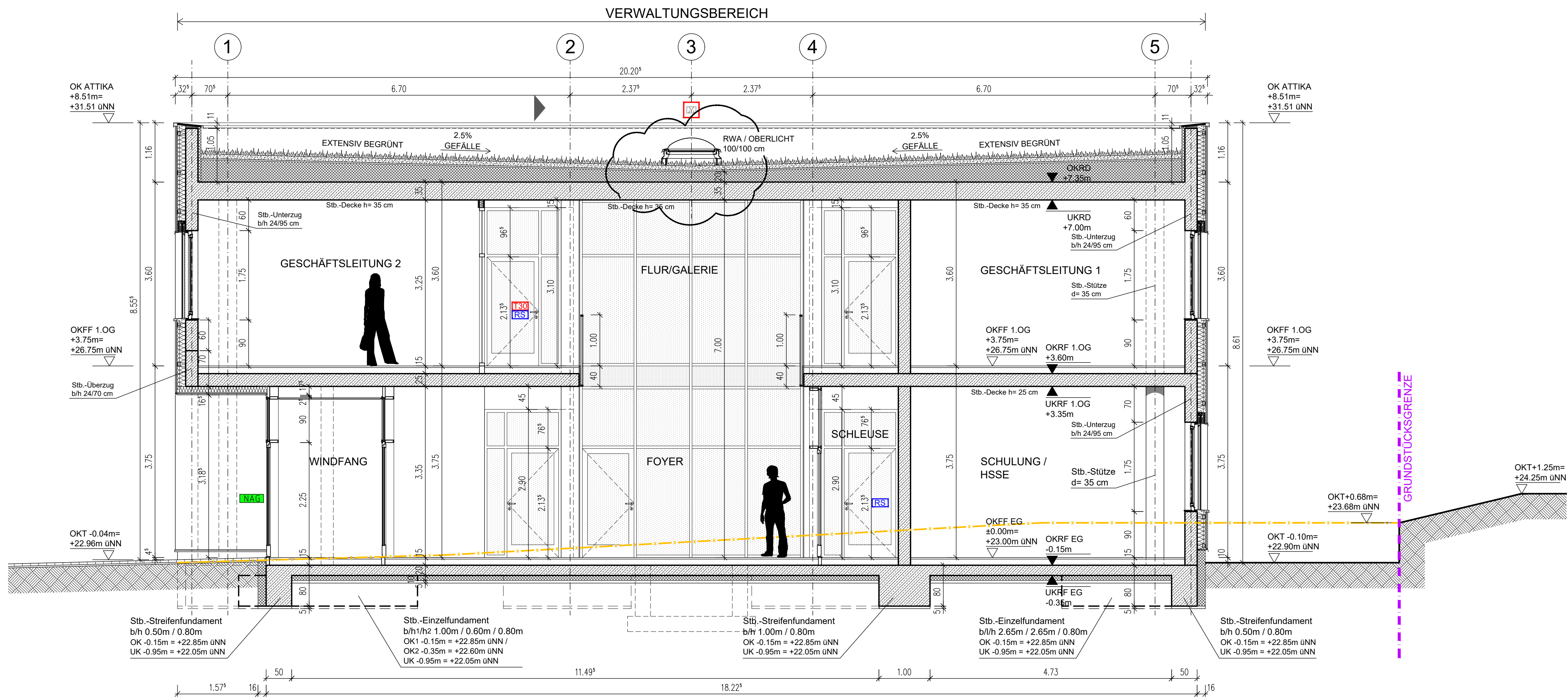
SNITT A-A
