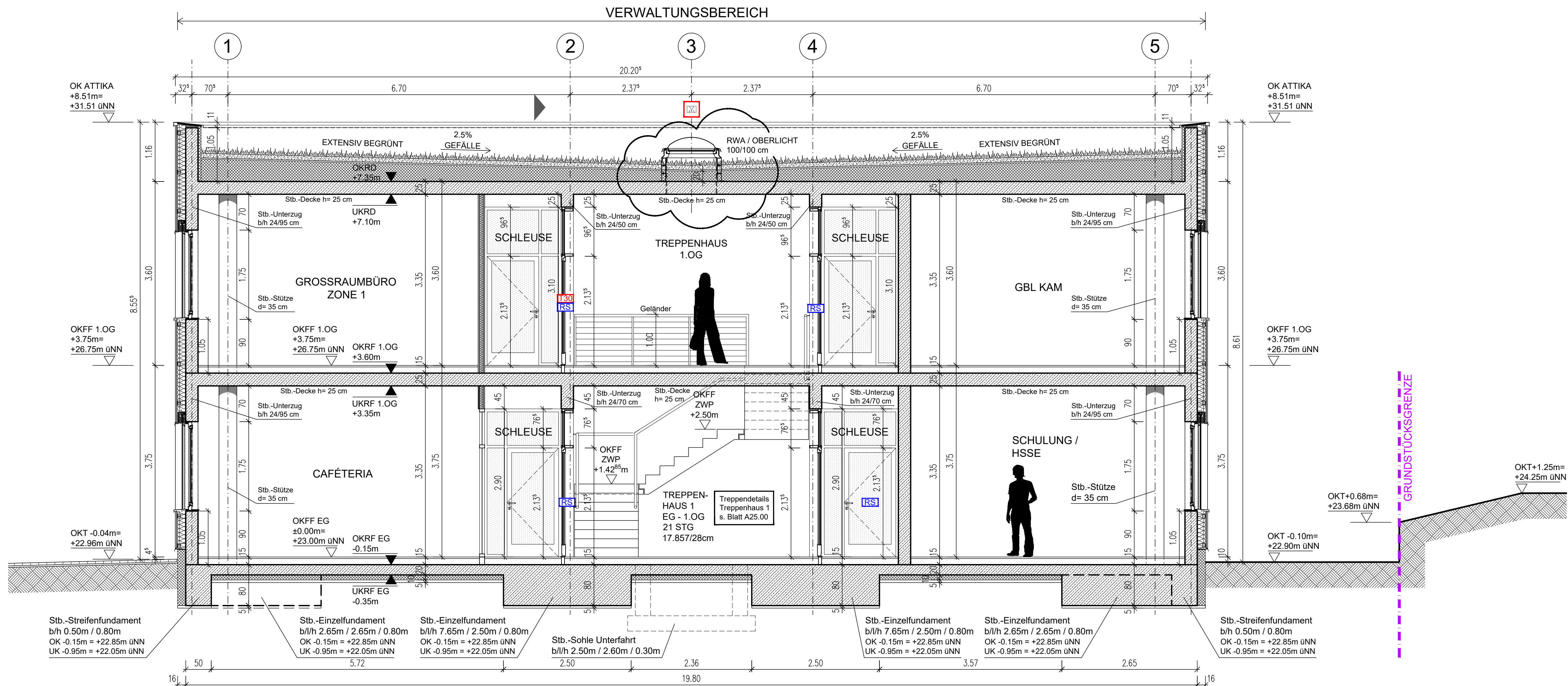
SNITT B-B
