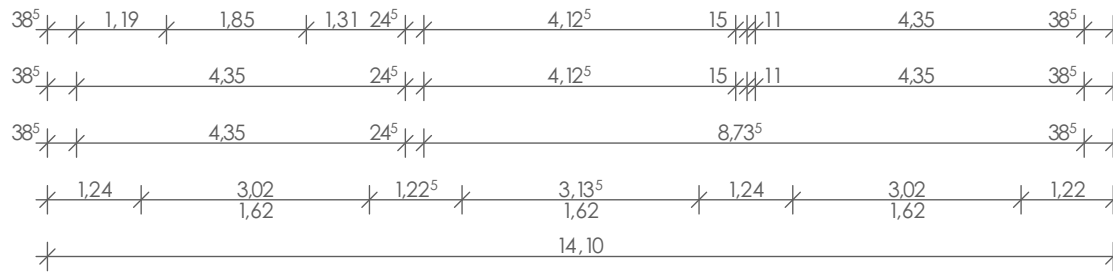
2. OBERGESCHOSS
