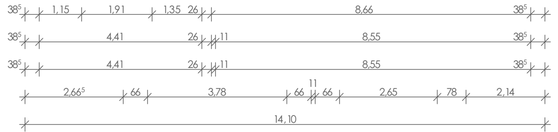
DACHGESCHOSS
