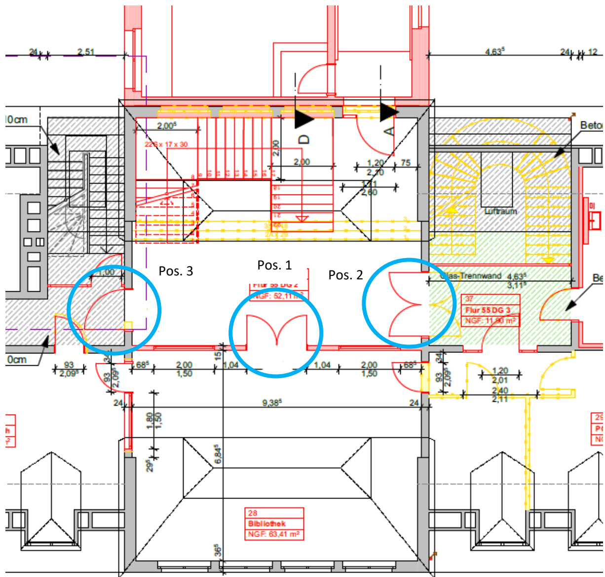
Abb.: Auszug Grundriss Dachgeschoss, Altbau 1955, GS Lüne
