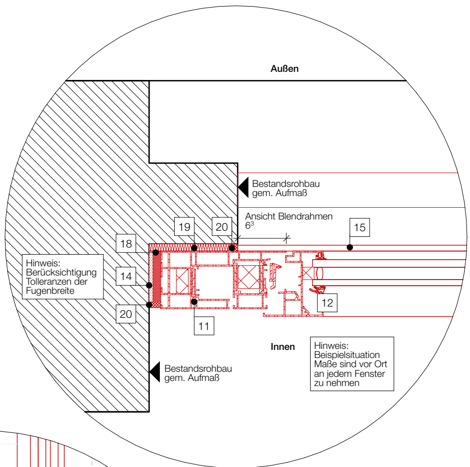
DETAIL Horizontalschnitt
