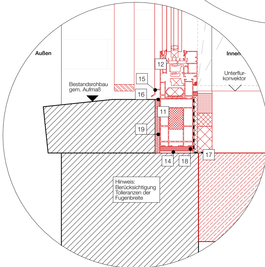
DETAIL Vertikalschnitt
