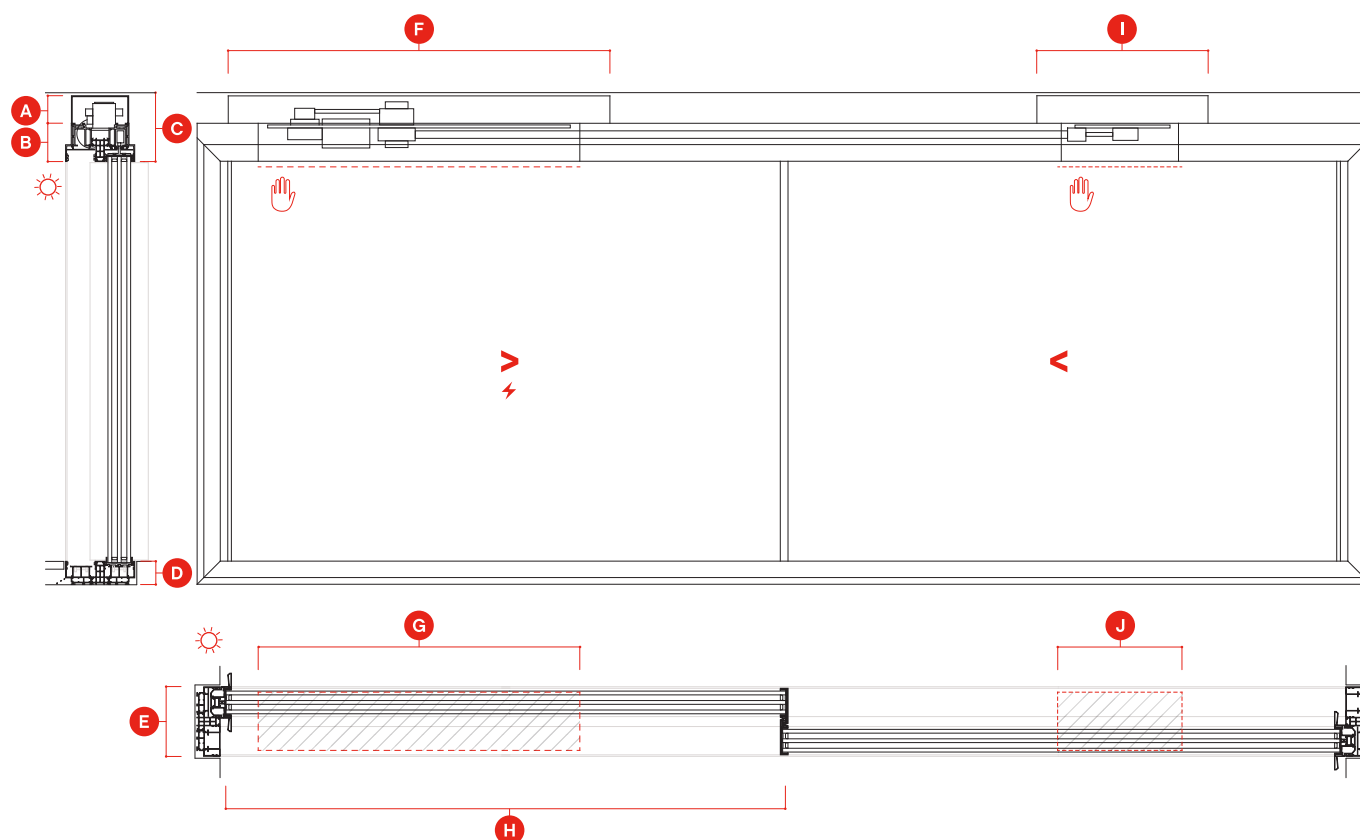
sliding birail horizontal section 2-schienige Horizontalschiebeanlage
